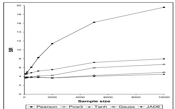
(d) GLD distributed source
